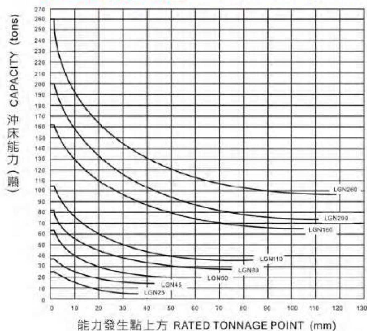
行程-能力曲線圖 Stroke - Capacity curve
